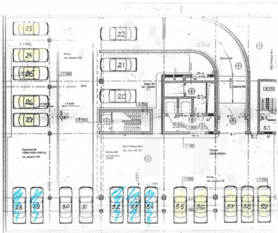
План паркинга
